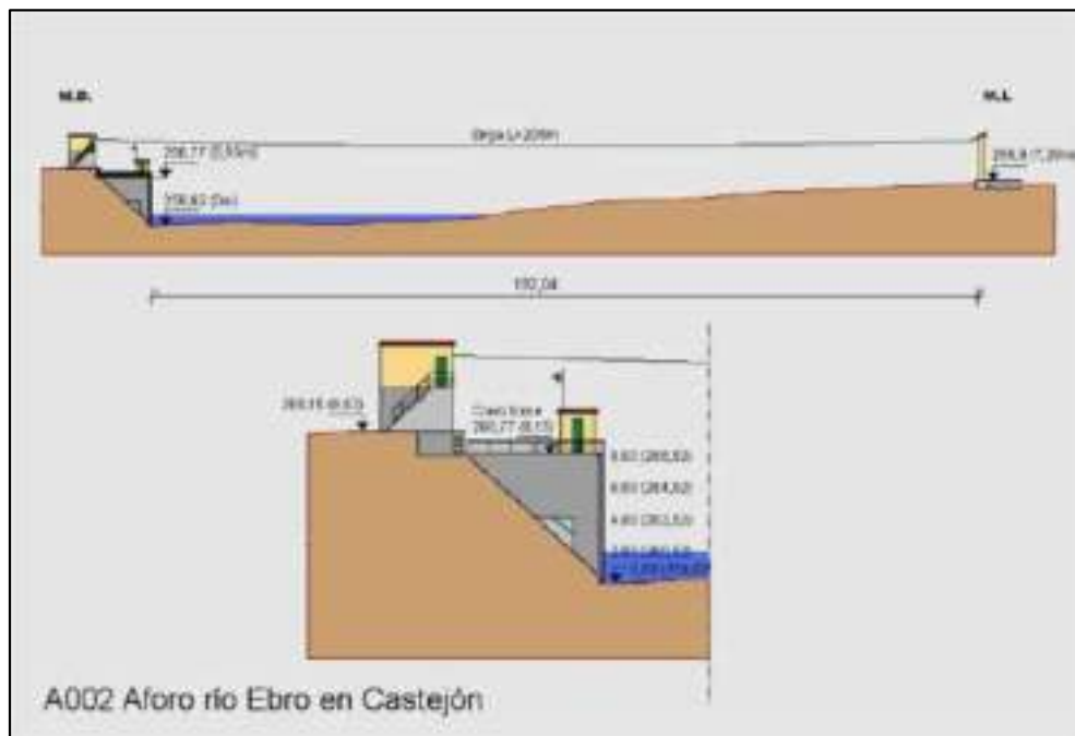
Ilustración 9. Esquema de medición de la sección de la estación de aforo de la CHE en el río Ebro en Castejón.
