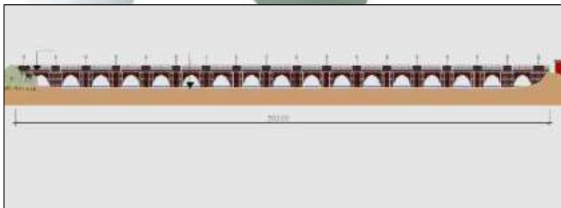
Ilustración 11. Esquema de medición de la sección de la estación de aforo de la CHE en el río Ebro en Tudela.
