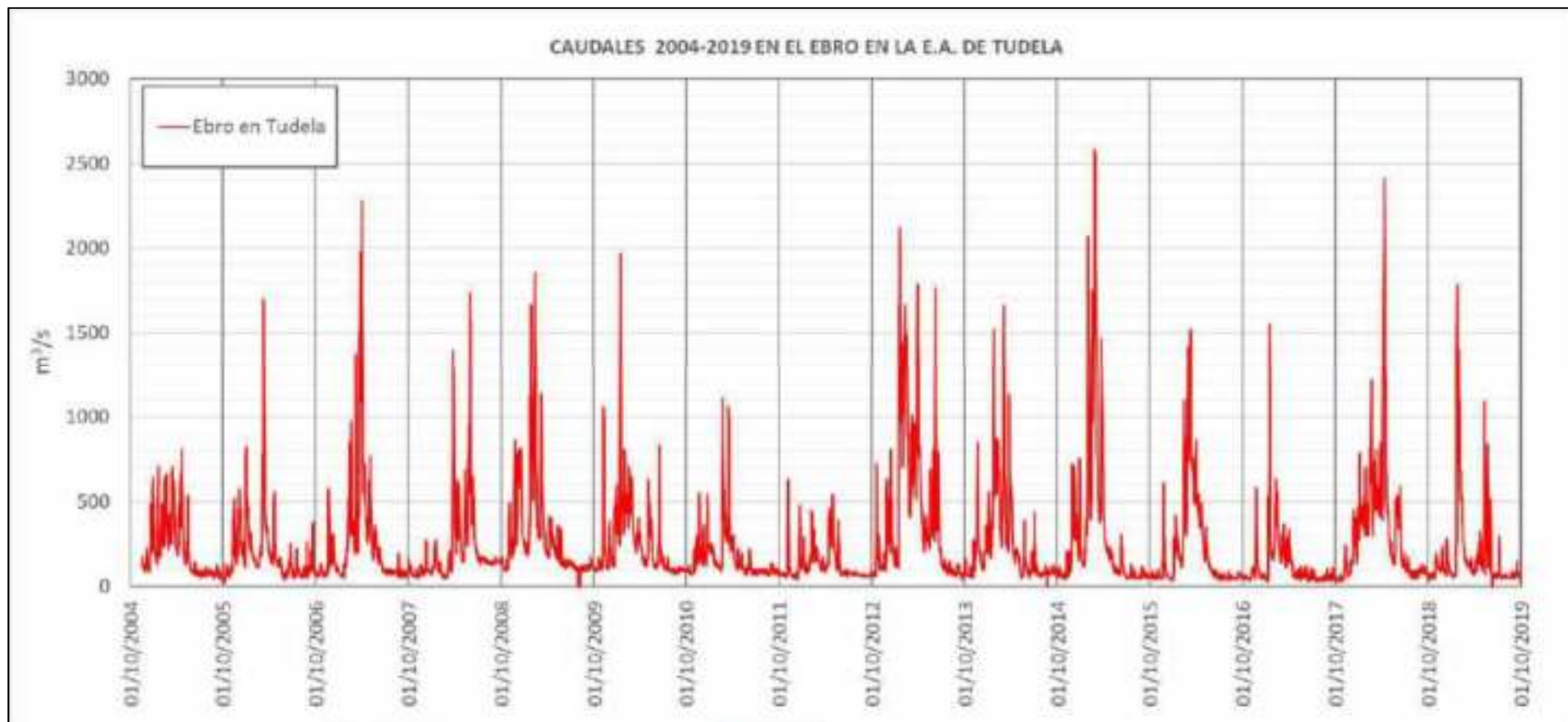
Ilustración 19. Valores máximos - instantáneos - diarios de los últimos 15 años hidrológicos (2004-2019), registrados en la estación de aforo del Ebro en Tudela (Obtenidos de la sección datos históricos de la CHE).
