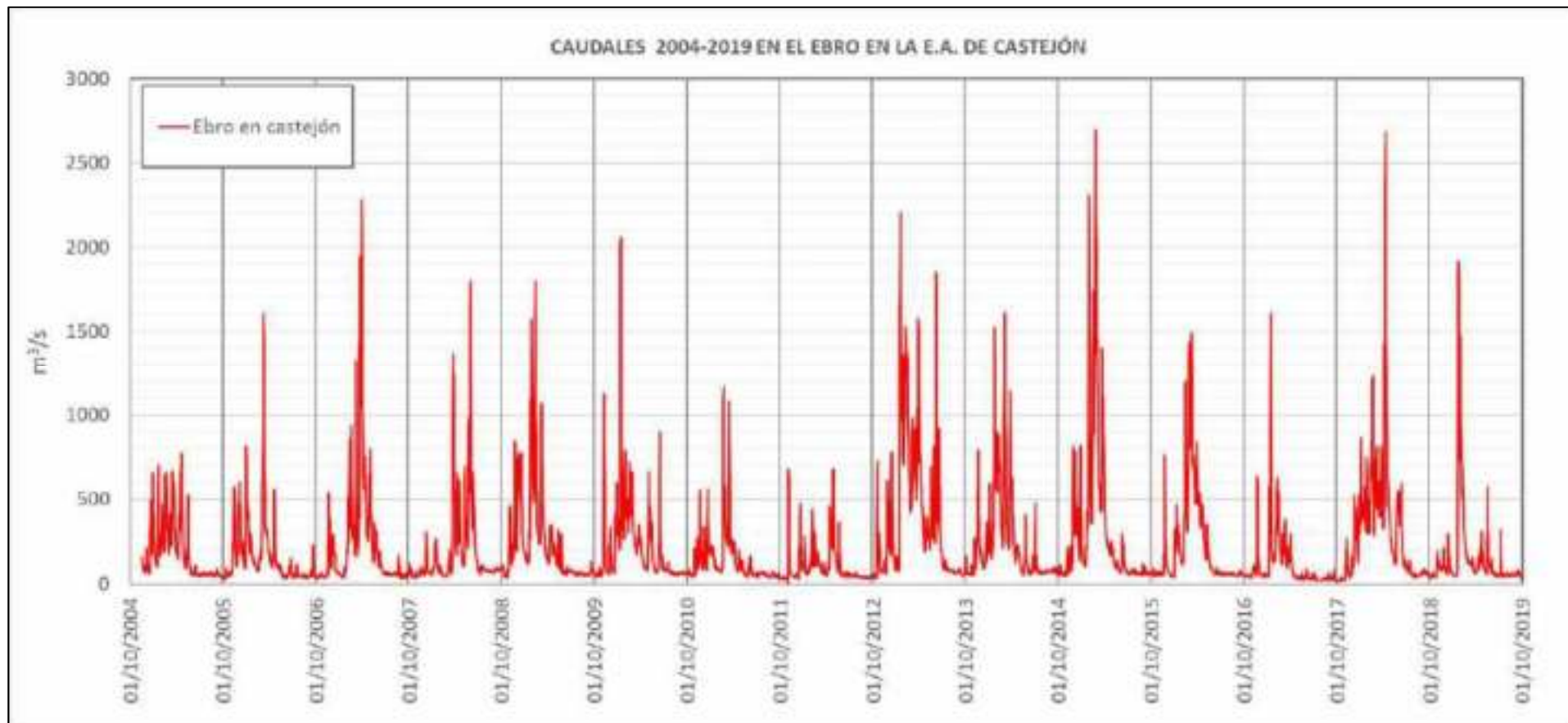
Ilustración 18. Valores máximos - instantáneos - diarios de los últimos 15 años hidrológicos (2004-2019), registrados en la estación de aforo del Ebro en Castejón (Obtenidos de la sección datos históricos de la CHE).
